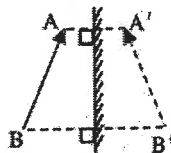
平面镜成像 A
